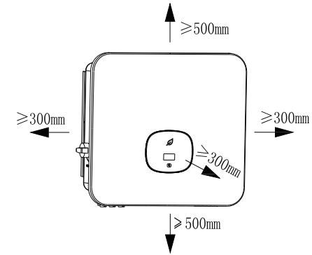
Fig 5.2 Dimensioni di installazione per un inverter
