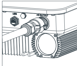
Fig 6.7 Schema di collegamento rapido AC
