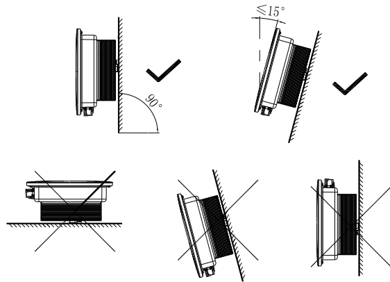
Fig 5.1 Schema di installazione
