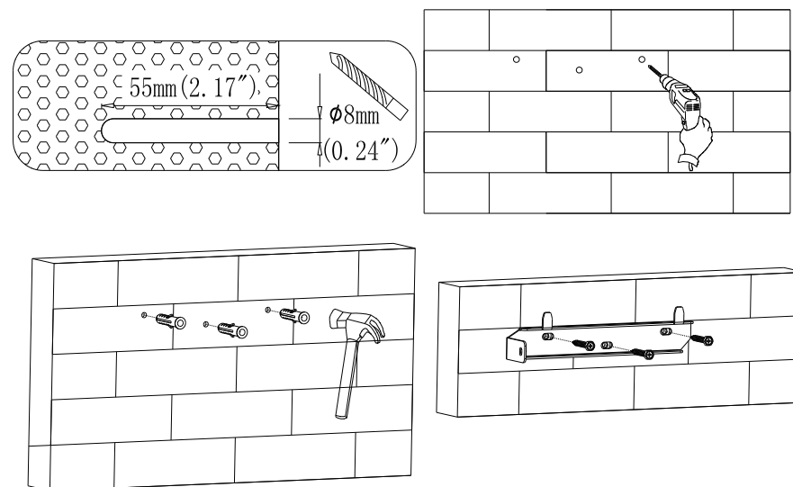
Fig 5.8 Schema del montaggio a parete
