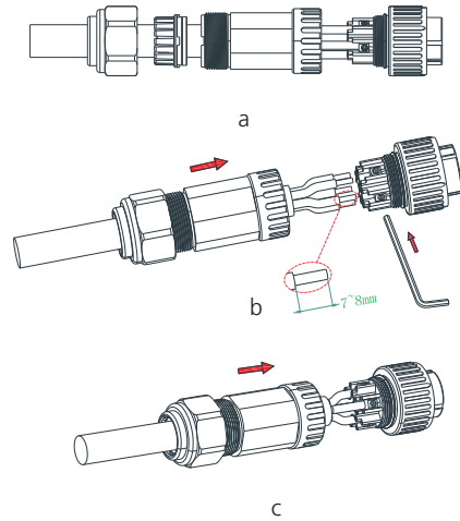
Fig 6.5 Schema di collegamento dell'uscita AC
