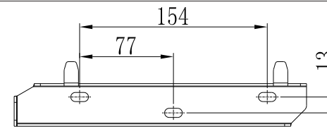
Fig 5.7 Specifiche del montaggio a parete
