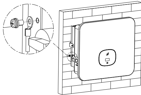
Fig 6.1 Diagramma di messa a terra
