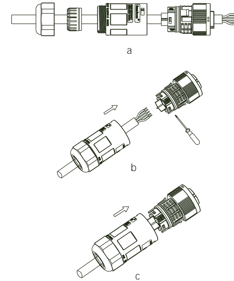
Fig 6.2 Schema di collegamento dell'uscita AC
