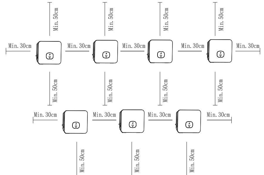
Fig 5.3 Dimensioni di installazione per più inverter
