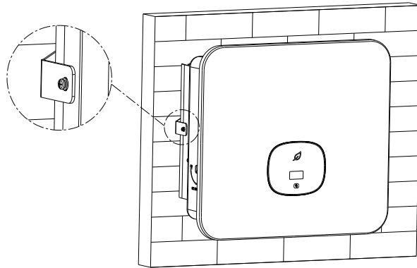
Fig 5.9 Schema del montaggio a parete dell'inverter
